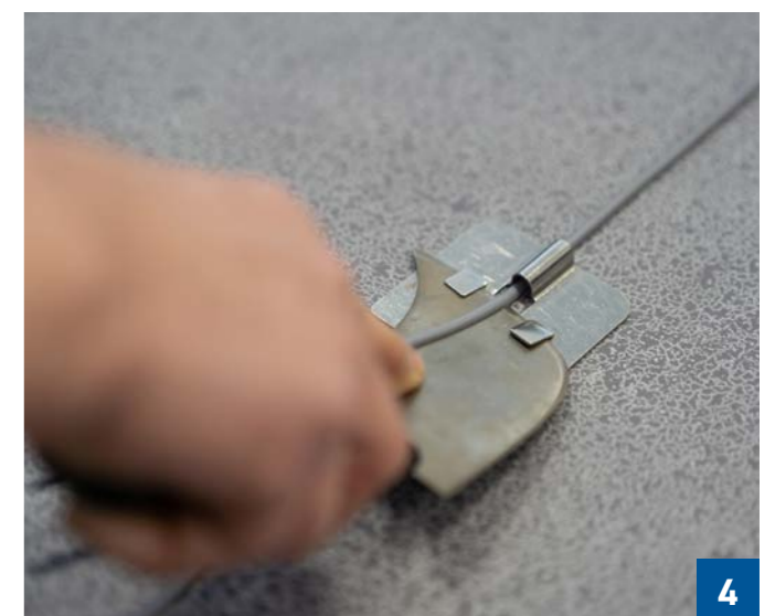
První seřezávání šňůry
