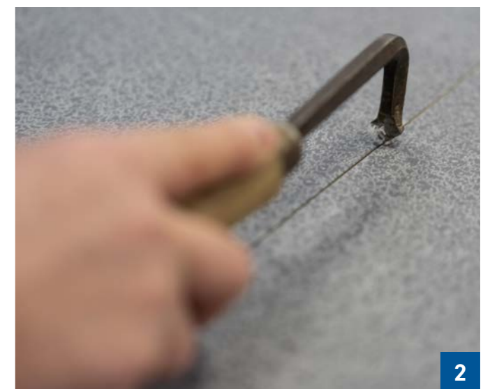
Drážkování před svařováním
